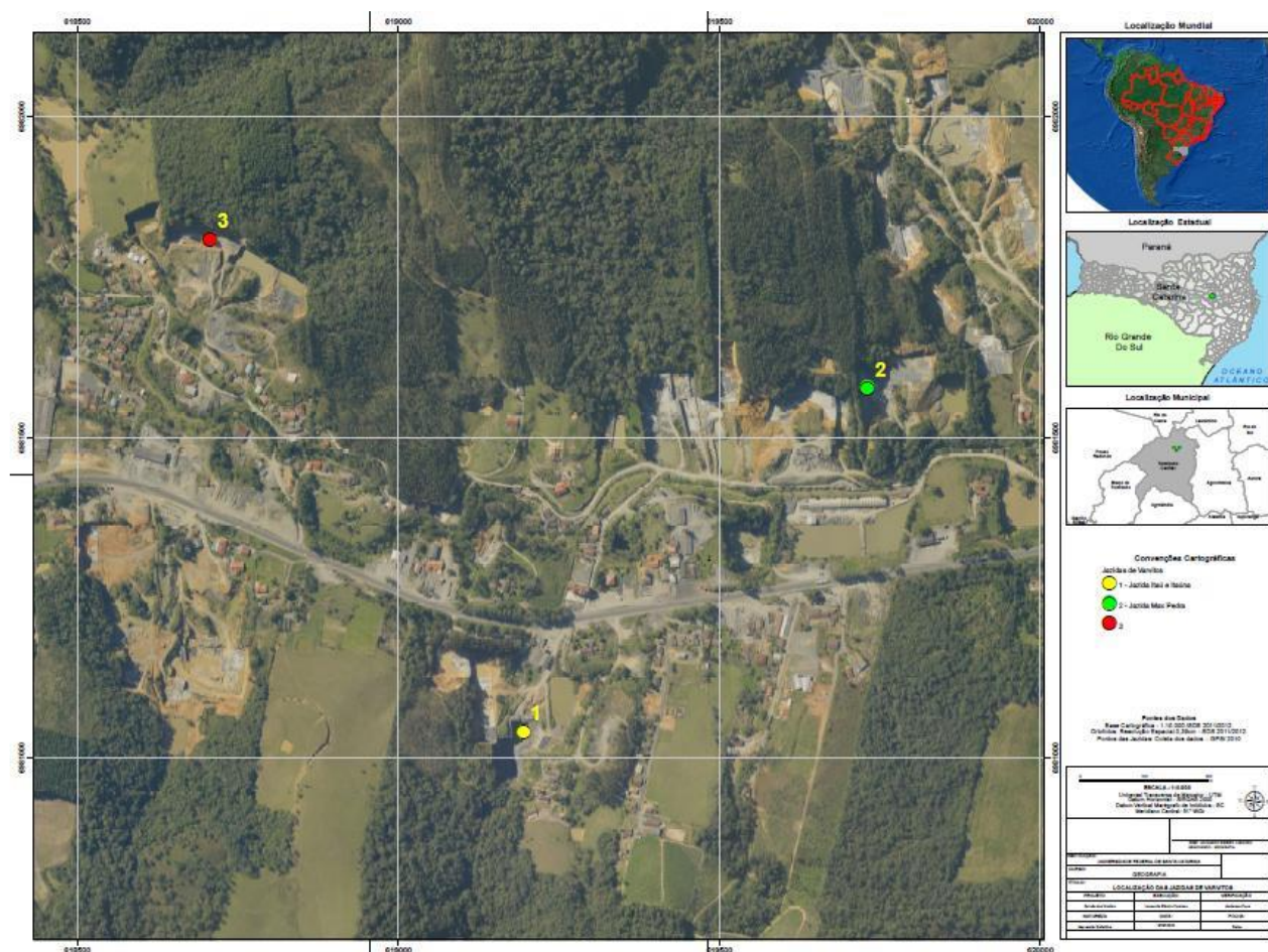
Figura 01. Localização dos três pontos de observação no município de Trombudo Central. Fonte: base cartográfica e orto-foto/SDS-SC/2012.
