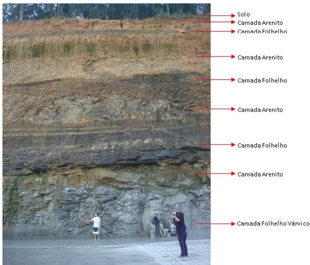
Figura 02. Exposição de rochas da Formação Rio do Sul. No corte observam-se as diversas camadas de rochas sedimentares, sobrepostas ao varvito. Localização: município de Trombudo Central/SC. Foto: Jéssica Santos (2010).
